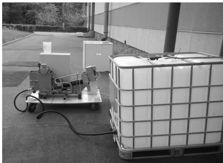
Рис. 6. Пилотная установка шнекового обезвоживателя «Аmson» серии ES-50
