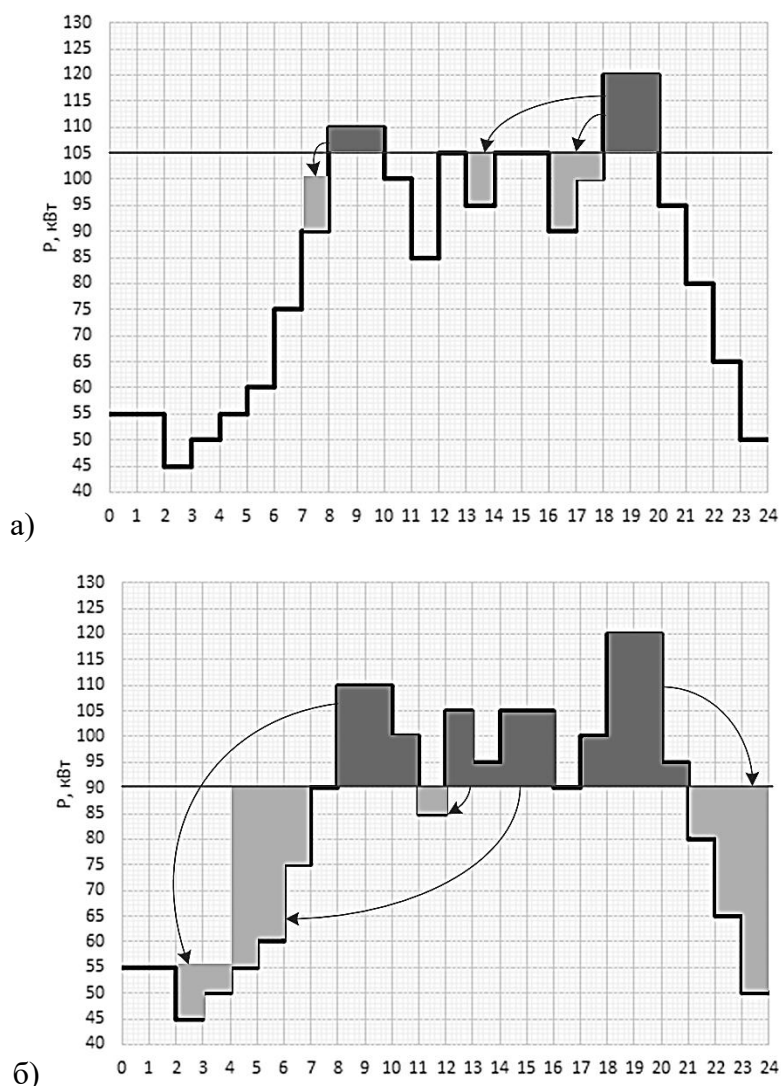
Рисунок 1 – Пример управления режимами энергопотребления при изменяющемся лимите мощности на АЭК: а) P_i = 105 кВт, б) P_i = 90 кВт
