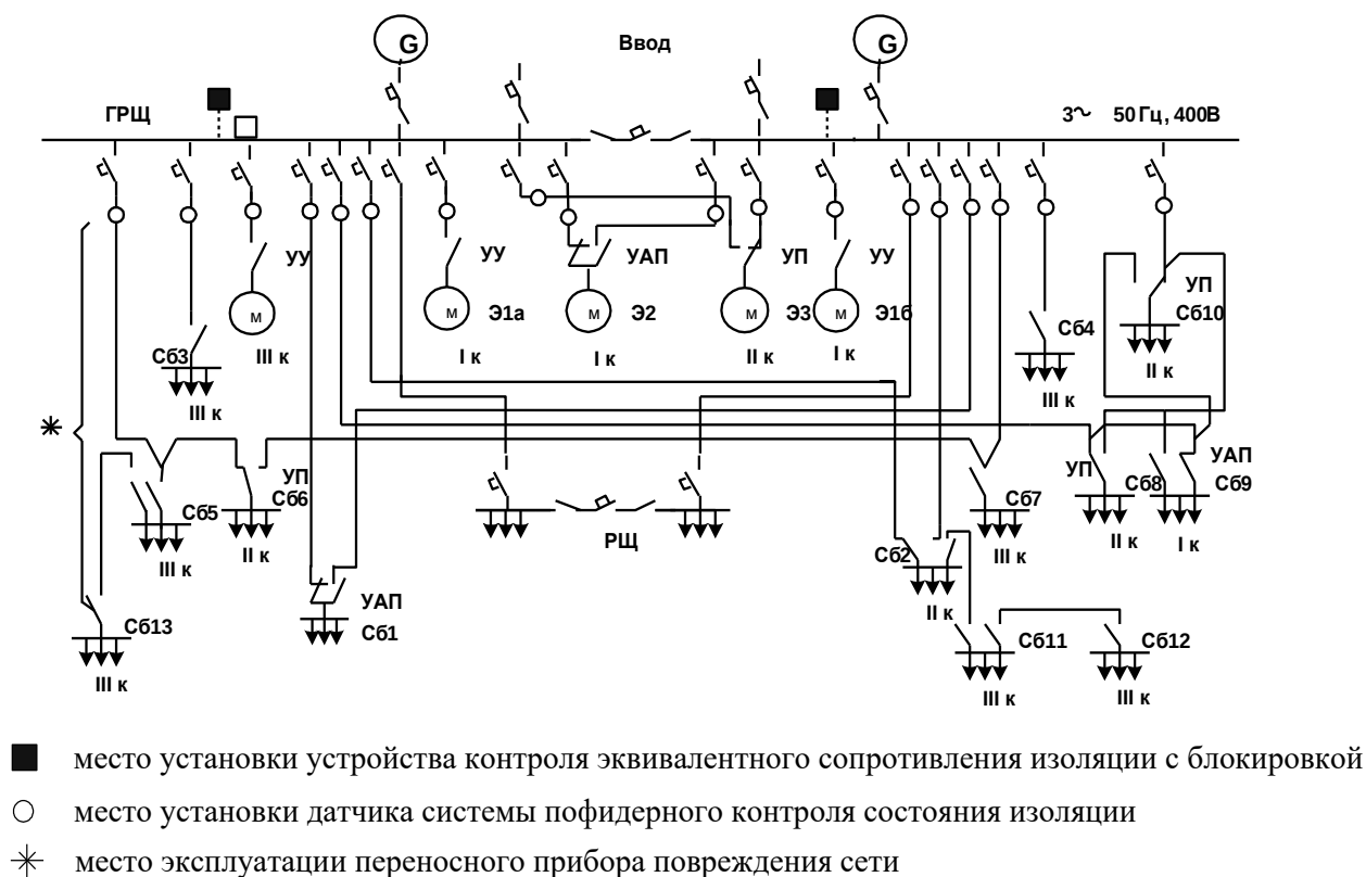
Рис. 2. Схема применения приборов контроля в СЭС 0,4кВ
