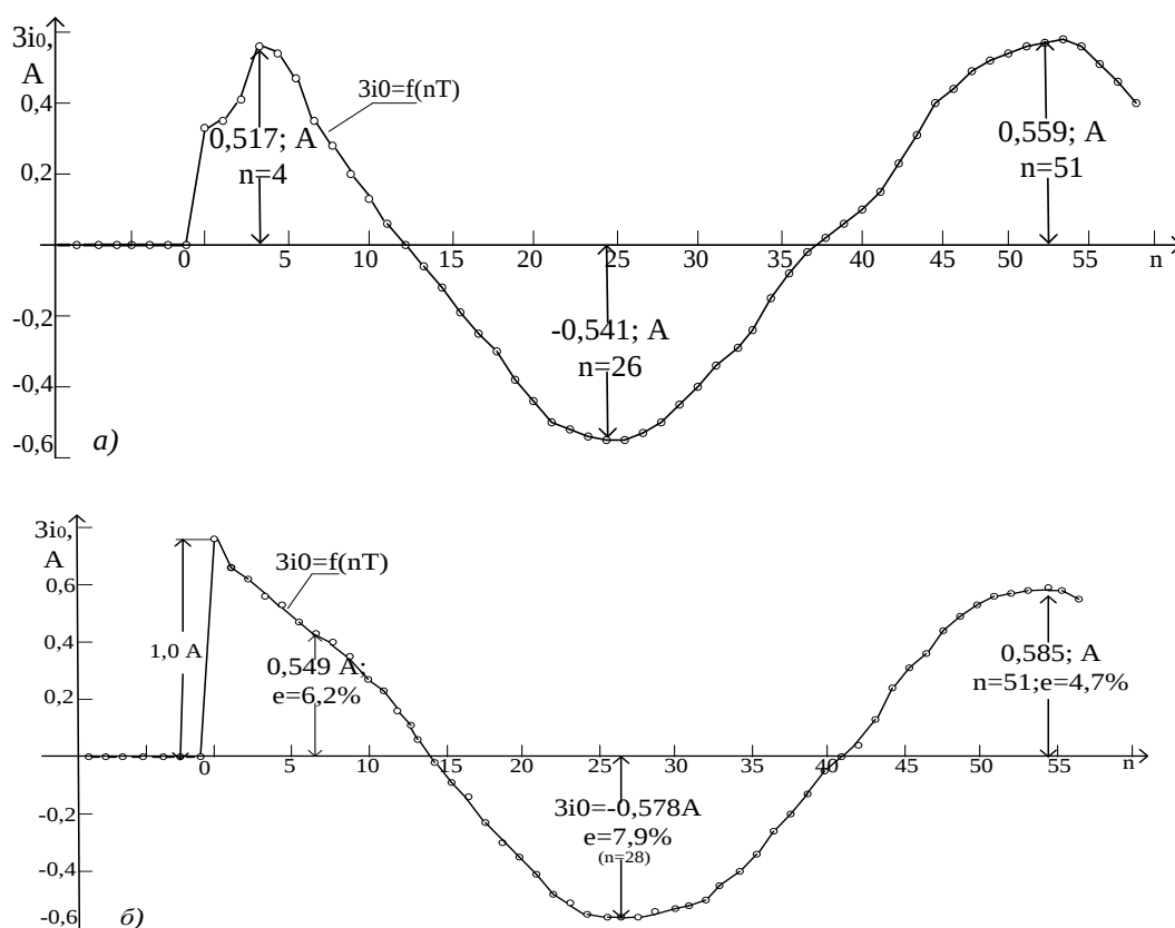
Рис. 3. Расчетные и опытные зависимости тока нулевой последовательности 3i_0 во времени 3i_0=f(nT) :
