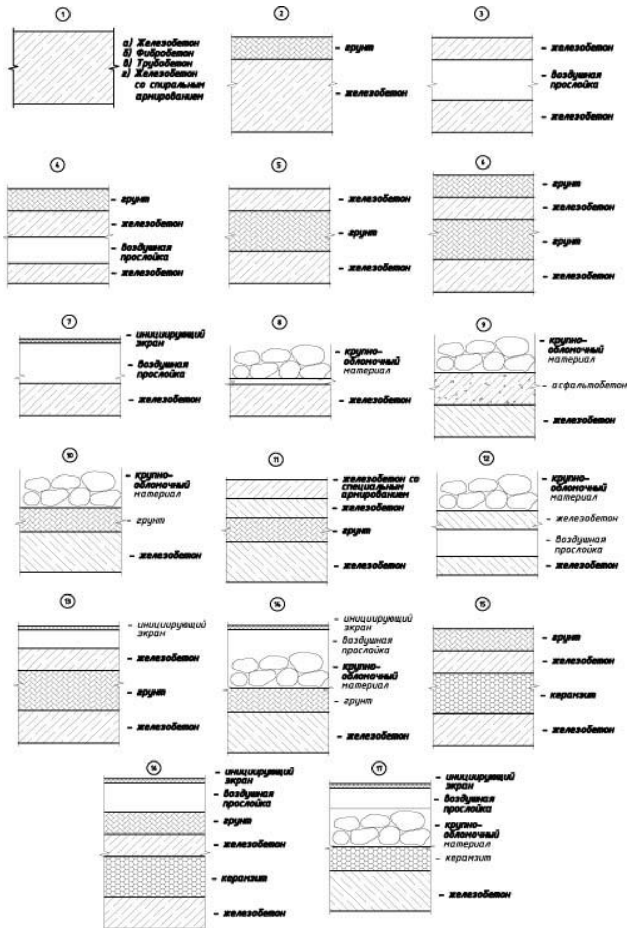
Рисунок 1. Конструкции энергопоглощающих и рикошетирующих туюфяков.
