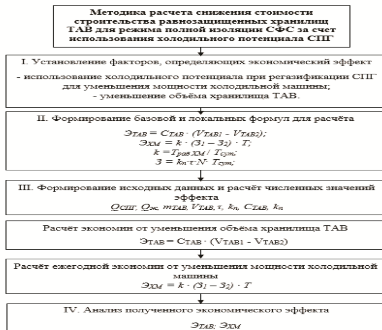
Рисунок 1. Блок-схема методики расчета снижения стоимости строительства хранилищ ТАВ для режима полной изоляции СФС за счет использования холодильного потенциала СПГ
