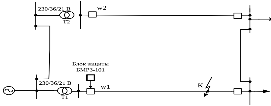
Рис. 2. Исходная схема ЭЭС
