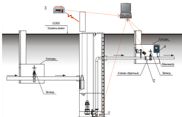
Рис.7. Система управления энергопотреблением при эксплуатации канализационных насосных станций.
