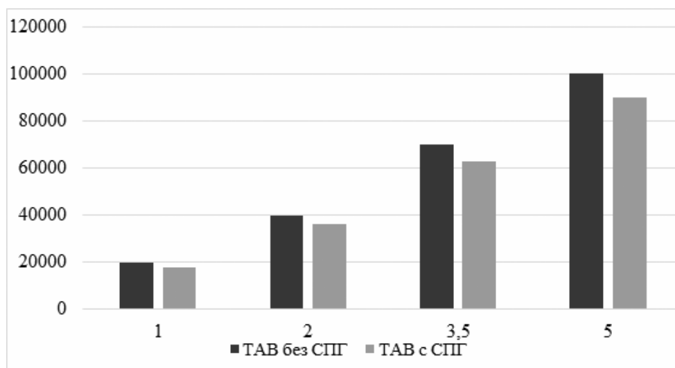
Рисунок 4. Уменьшение объёма ТАВ за счёт холодильного потенциала СПГ
