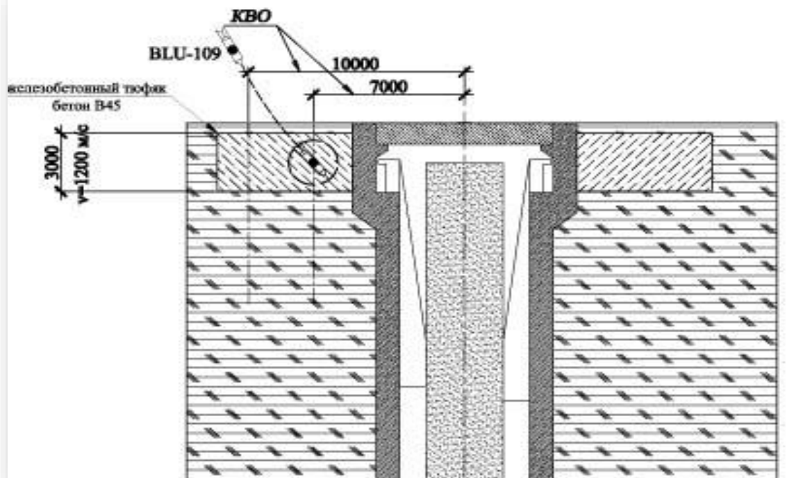
Рисунок 2. Определение толщины железобетонного туюфака
