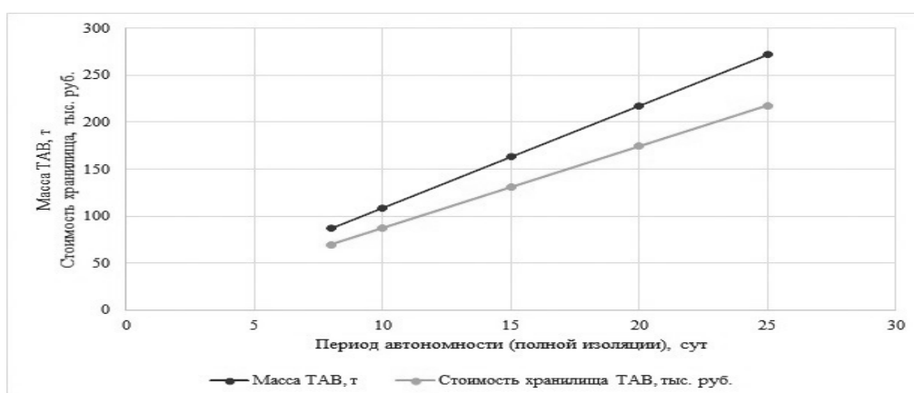
Рисунок 3. Изменение количества ТАВ и стоимости строительства хранилища ТАВ в зависимости полной изоляции
