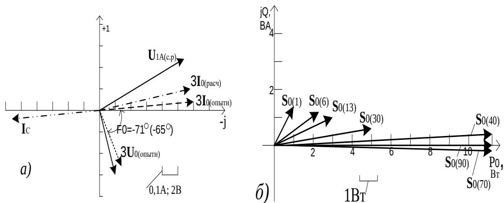
Рис. 4. Векторные диаграммы величин режима ОЗЗ фазы 3(С): а – расчетные и опытные значения 3I_0 , 3U_0 , I_c для момента времени nT=0,012 с ( n=28 ); б - изменение действительных координат вектора S_0 во времени ( S_0=f(nT) ) от момента коммутации S^{(1)}_0 ( n=0 )( t_0 ) до n=100 ( t=0,0417 с.).
