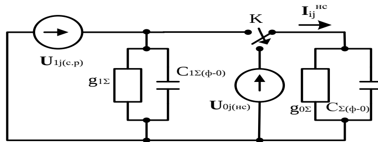
Рис. 1. Эквивалентная схема замещения ЭЭС для точки коммутации К
