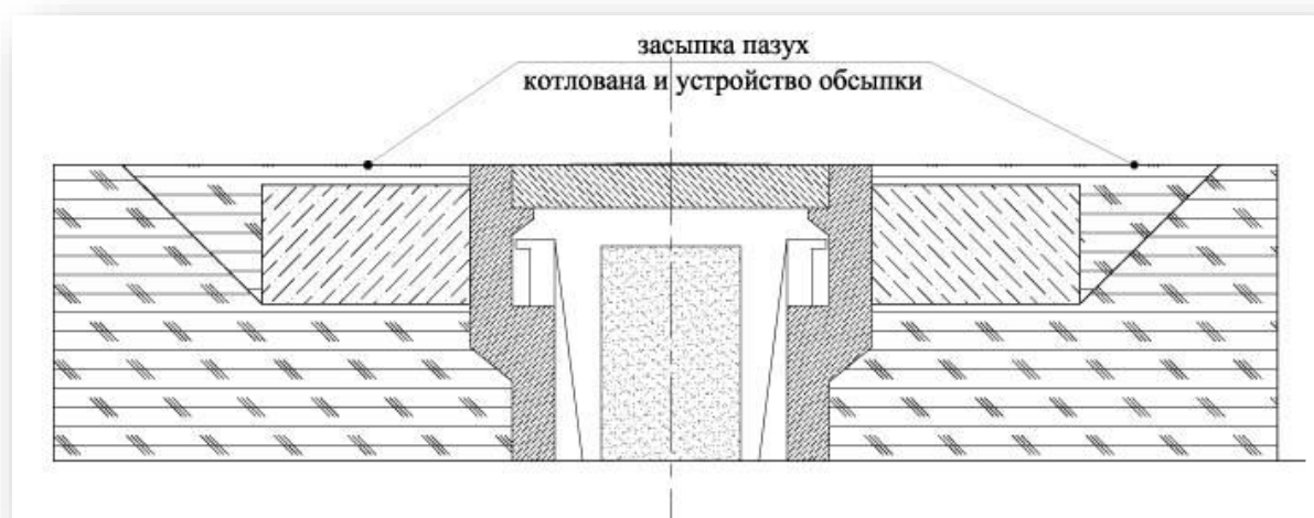
Рисунок 5. Устройство железобетонного тюфяка
