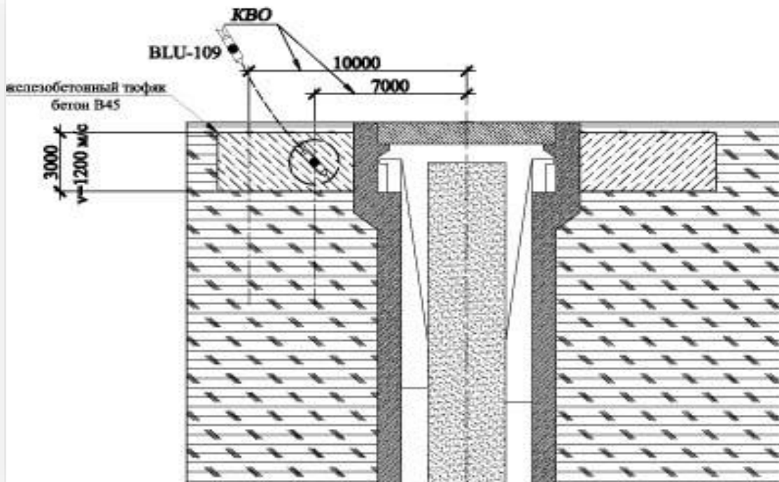
Рисунок 2. Определение толщины железобетонного туюфака
