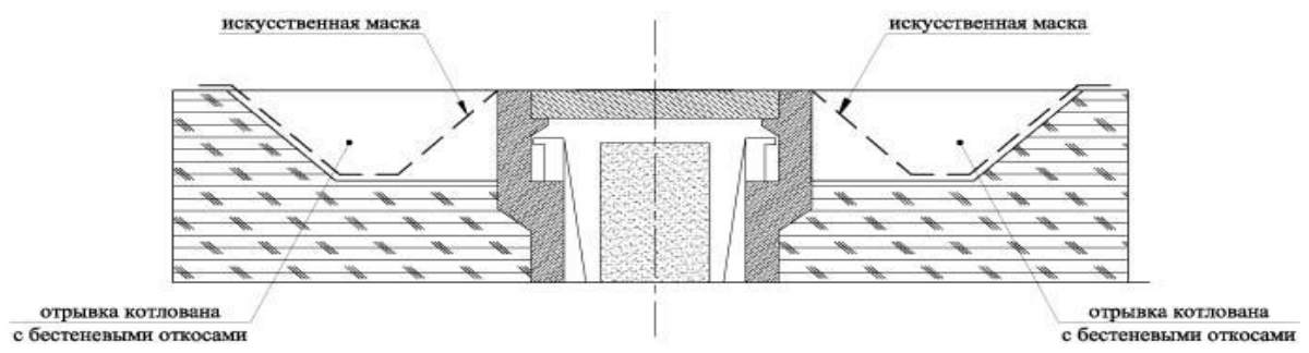
Рисунок 2. Определение толщины железобетонного туюфака
